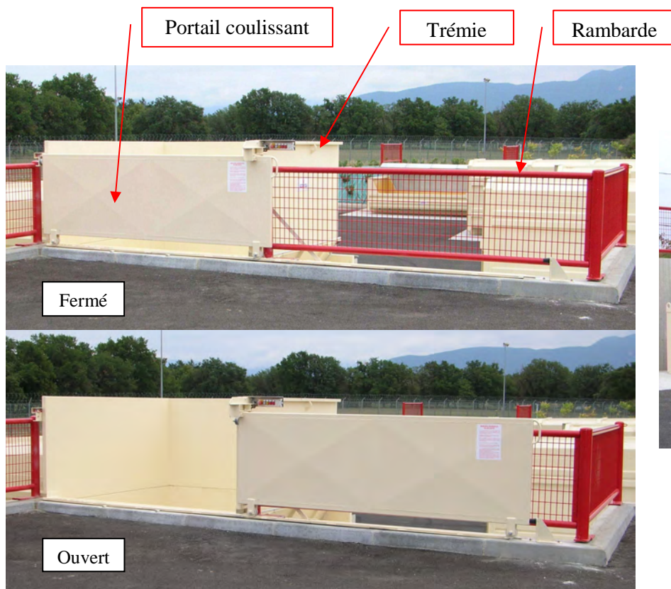
Portail de sécurité coulissant devant la trémie (vue du quai)
